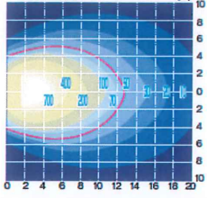
■水平面照度分布図(ルクス) ※マスト最大高さ2.6mで灯具角度-30°の場合
