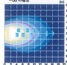
■水平面照度分布図(ルクス) ※マスト最大高さ2.2mで灯具角度-30°の場合
