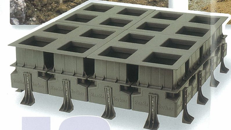
ビー・ビー・ワーカー [16型] 仕様 ● 材質 / ABS樹脂 ● サイズ / 108×108×28cm ● 重量 / 約20Kg
