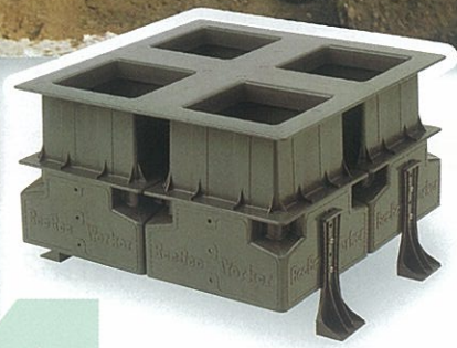
ビー・ビー・ワーカー [4型] 仕様 ● 材質 / ABS樹脂 ● サイズ / 54×54×28cm ● 重量 / 約5Kg
